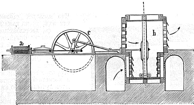
Рудничный поршневой вентиляторъ системы Никсона. Поршень h движется въ моментъ изображенія на рис. съ лѣва на право, а потому высасываніе идетъ изъ лѣваго устья, какъ видно по положенію клапановъ.
