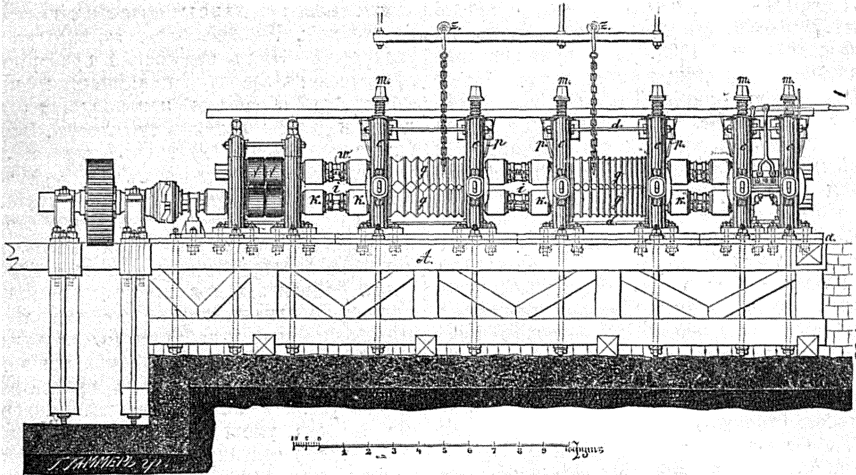
Фиг. 1. Прокатный станъ для полученія сортового желѣза (и стали). Общій продольный видъ.
