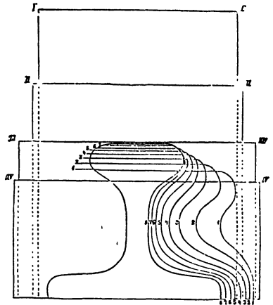
Фиг. 5. Послѣдовательное суженіе пакета при прокаткѣ рельсового желѣза (и стали).
