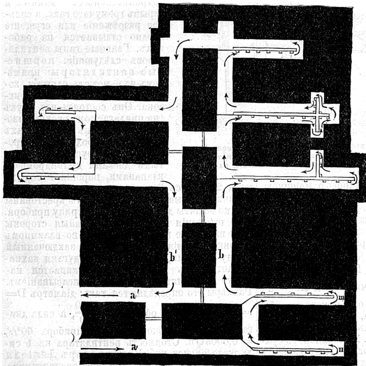
Способъ вентилярованія наменноугольныхъ копей, выдѣляющихъ гремучій газъ. Воздухъ, входящій въ a заставляеть, при помощи перегородокъ n , m и т. п., проходить во всѣ мѣста работы. Стрѣлки показывають ходъ воздуха, выходящаго изъ a' .
