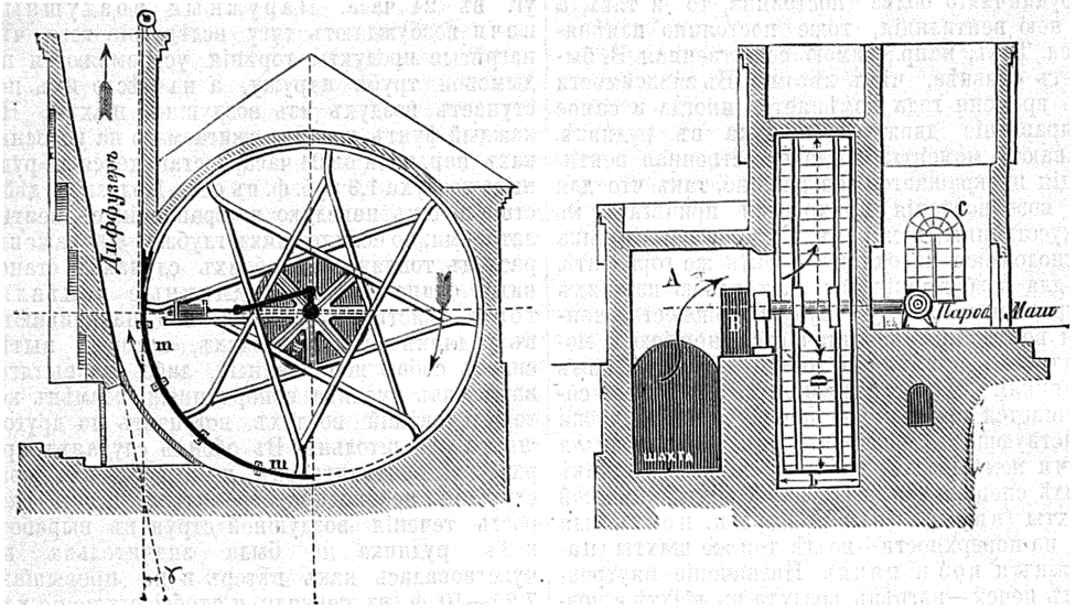
Центробѣжный рудничный вентиляторъ системы Габаля въ вертикальномъ разрѣзѣ, съ лѣва—перпендикулярно ось вращения, а съ праваяго по ней. Воздухъ движется отъ оси на окружности и уходитъ чрезъ диффузаръ.
